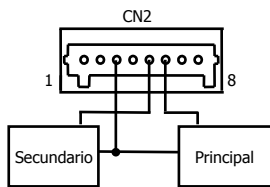
CAPTADOR NAMUR
