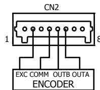
ENCODER
