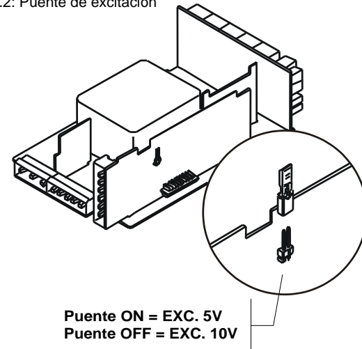
Fig. 16.2: Puente de excitación
