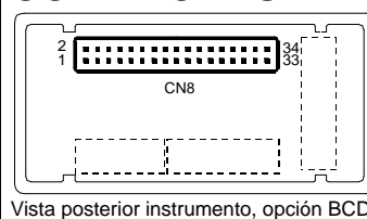
Vista posterior instrumento, opción BCD
